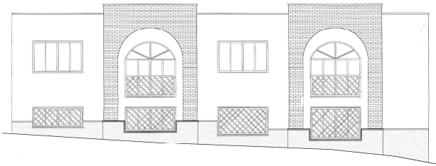
ALZADO A CAÑADA DEL RIO
